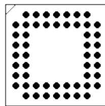
LCC-SKT52
