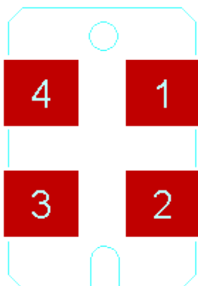
SOT227
