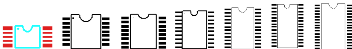
TSSOP10
