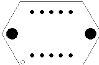
APEX-PD10
