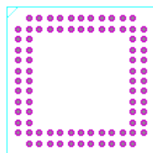
LCC-SKT84
