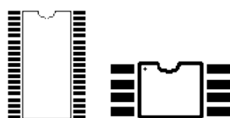
TSSOP38
