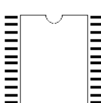
MO-019/24
