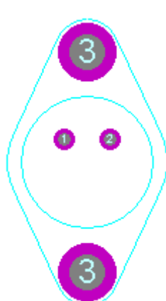
TO66
