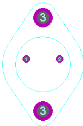
TO204
