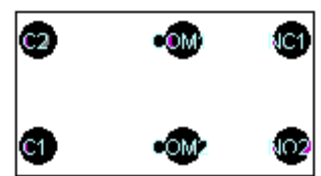
RLY-OMRON-G68-A3
