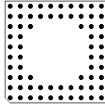
PGA68
