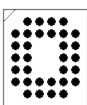
LCC-SKT32
