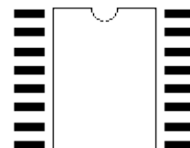
MO-004/16
